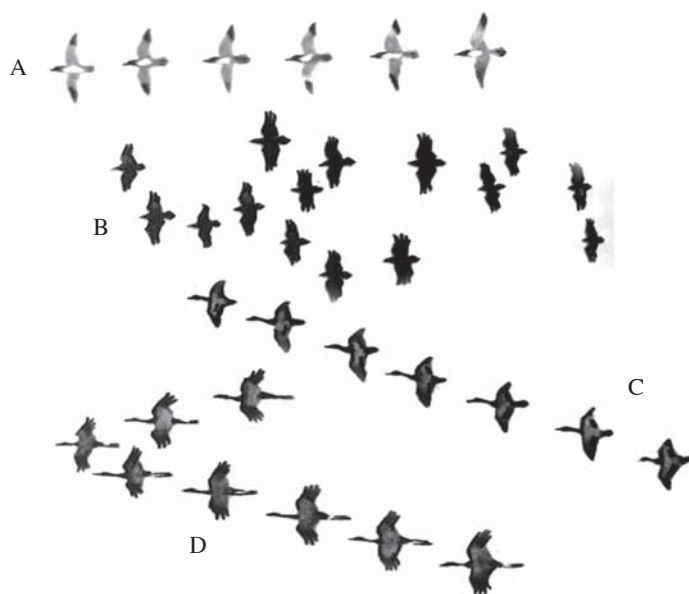
Siluety migrujících hejn (létají v klínu, aby se střídali při prorážení vzduchu, tak šetří energii). Formace hejna racků (A) a havranů (B), formace kachen (C) a formace hejna jeřábů (D).
